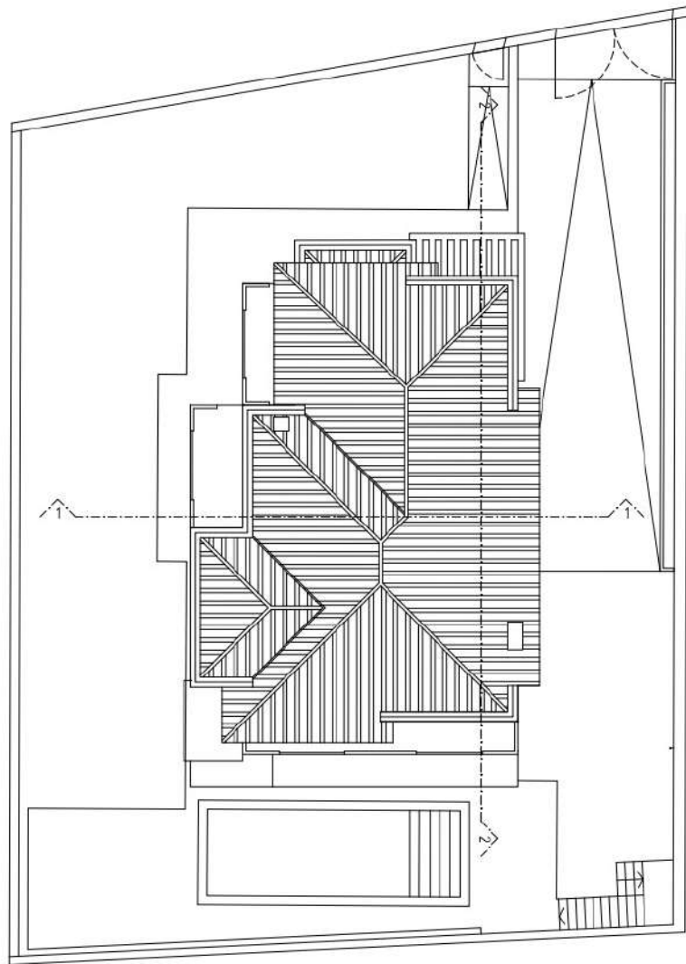
PLANTA COBERTURA Esc. 1:100
