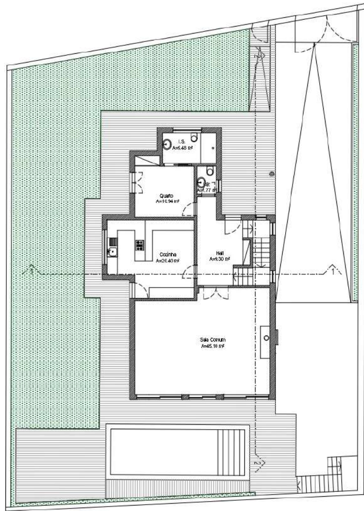
PLANTA PISO TÉRREO Esc. 1:100
