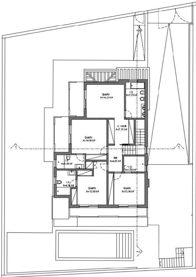
PLANTA PISO 1 Esc. 1:100
