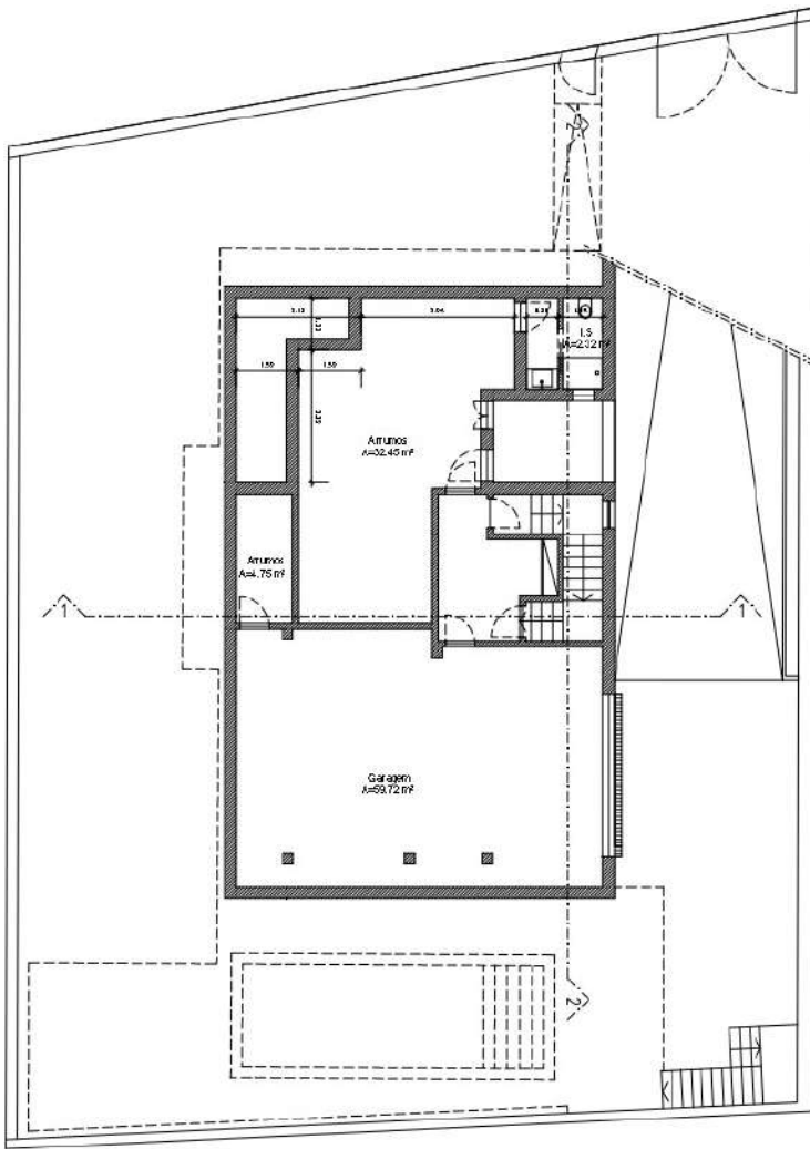
PLANTA PISO CAVE Esc. 1:100
